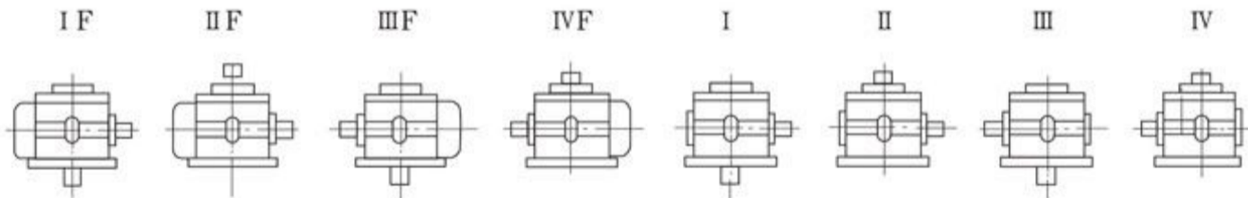
装配型式K向F-带风扇
