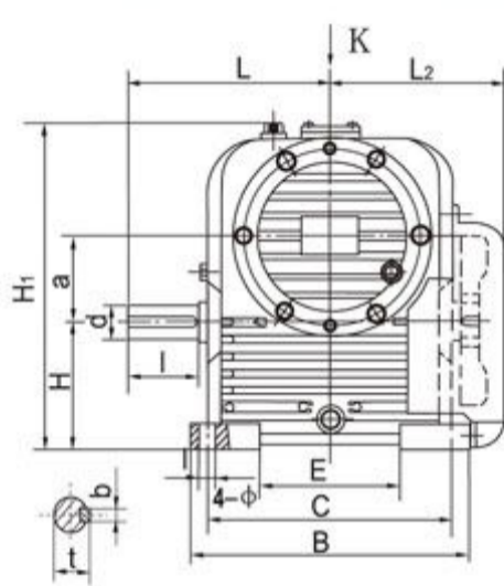
TPU型减速器（整箱式）及装配型式
