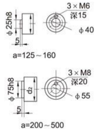
Ⅲ、ⅢF、Ⅳ、ⅣF带控制器用轴端
