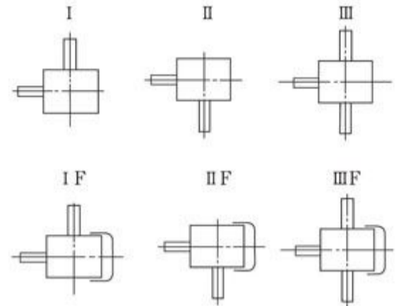
装配型式 (K向)
