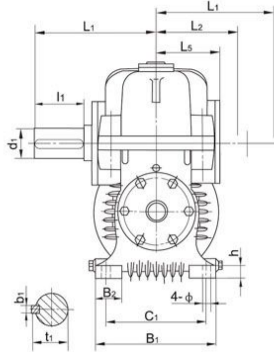
Ⅲ、ⅢF、Ⅳ、ⅣF带控制器用轴端
