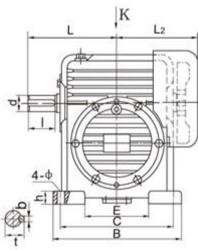
TPA型减速器（整箱式）及装配型式
