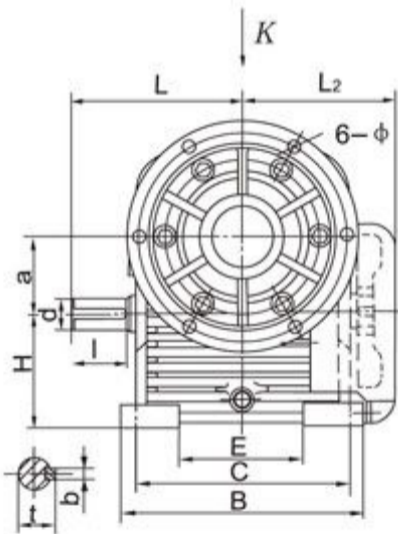
TPS型减速器（整箱式）及装配型式
