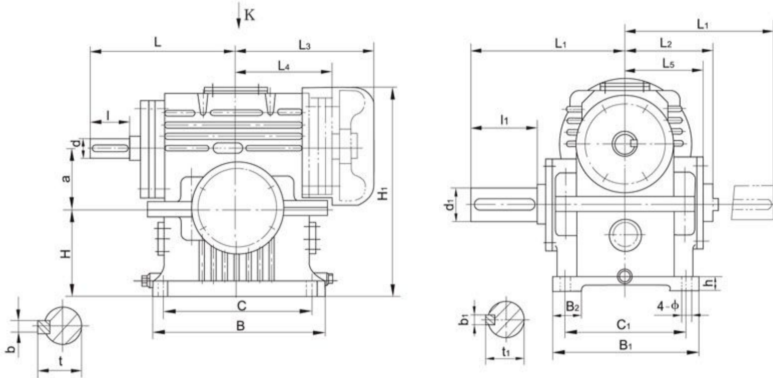
装配型式K向F-带风扇
