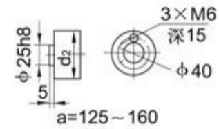
Ⅲ、ⅢF、Ⅳ、ⅣF带控制器用轴端
