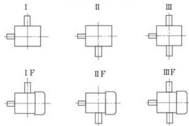
装配型式(K向)
