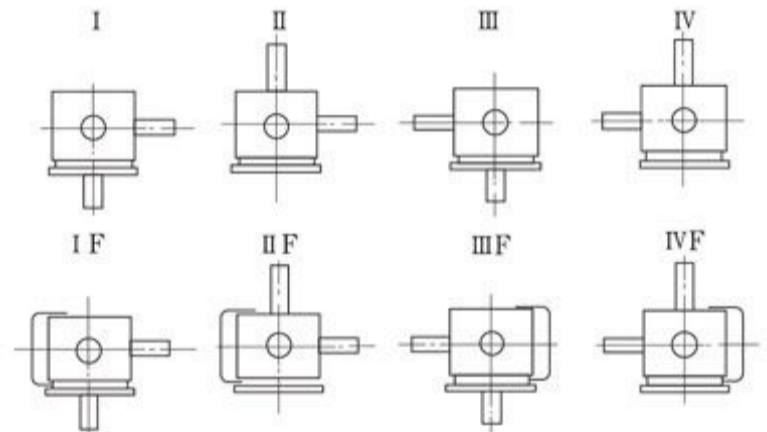
装配型式(K向旋转)
