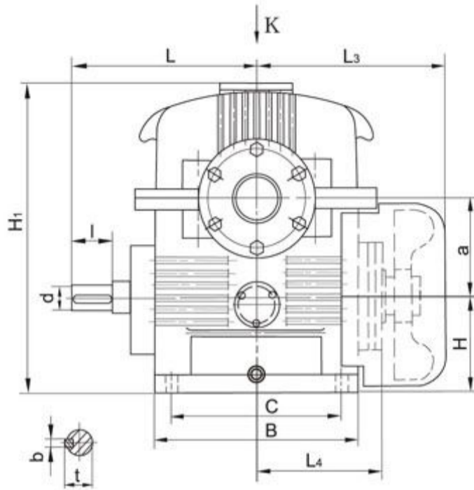
装配型式K向F-带风扇
